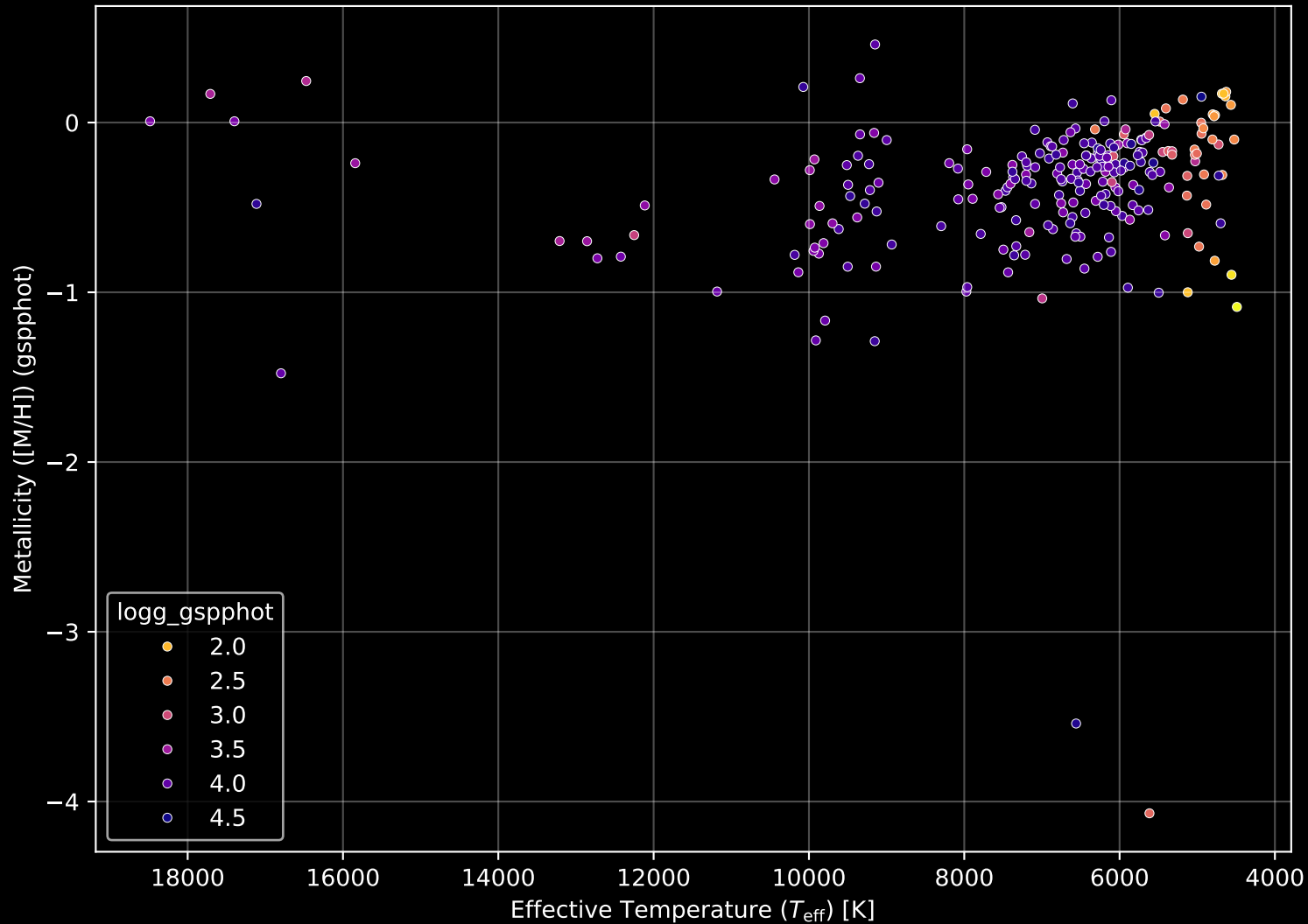
GALAH DR4 Field: [9222] Stellar Population Parameters (n= 245)
