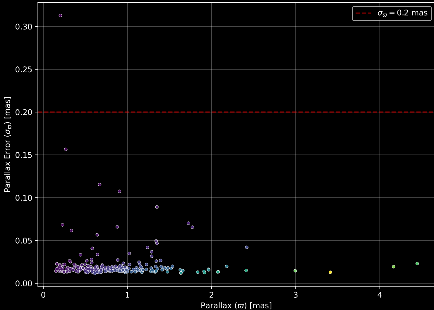
GALAH DR4 Field: [9222] Parallax Quality (n= 245)
