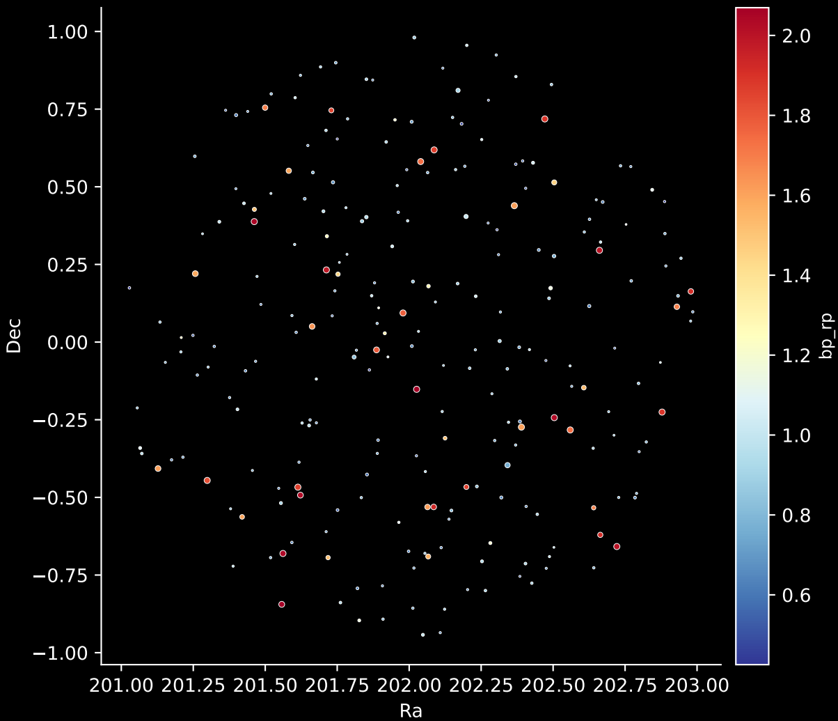
GALAH DR4 Field: [9222] Stars: 245
