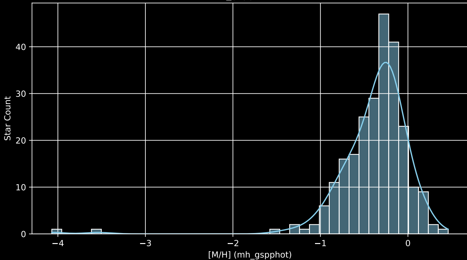
GALAH DR4 Field: [9222] [M/H] (mh_gspphot) (n= 245)
